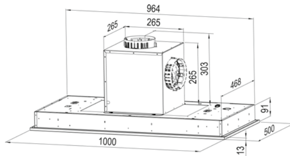
Deckenhaube Modula mit Motorgruppe
