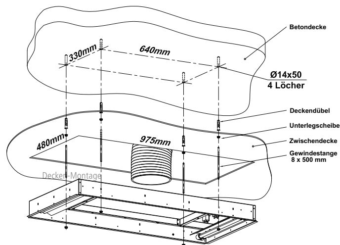
Empfohlener Mindestabstand über Elektrokochstelle/Gaskochstelle: 90 cm
