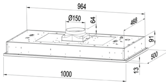
Deckenhaube Modula ohne Motorgruppe
