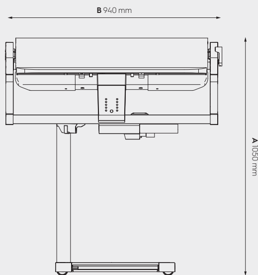
Seitenansicht
